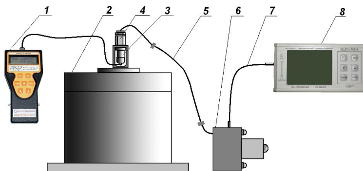
1 – измеритель параметров вибрации; 5 – удлинитель; 2 – виброгенератор; 6 – датчик силы ПДУ; 3 – датчик измерителя параметров вибрации; 7 – кабель прибора; 4 – акселерометр; 8 – электронный блок ПДУ.
